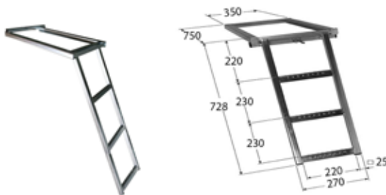
Escalera bajo-chasis de 3 peldaños (750 mm.) modelo "E"
